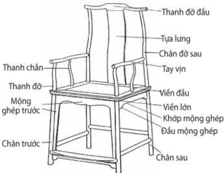
Sơ đồ cấu tạo của chiếc ghế tựa mũ quan.
